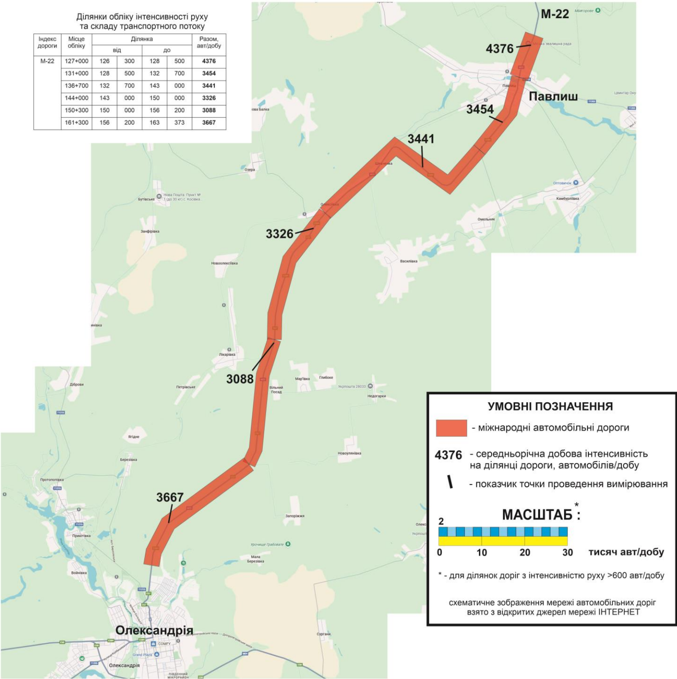
Епюра середньорічної добової інтенсивності руху на основних перегонах автомобільної дороги М-22 Полтава-Олександрія у Кіровоградській області
