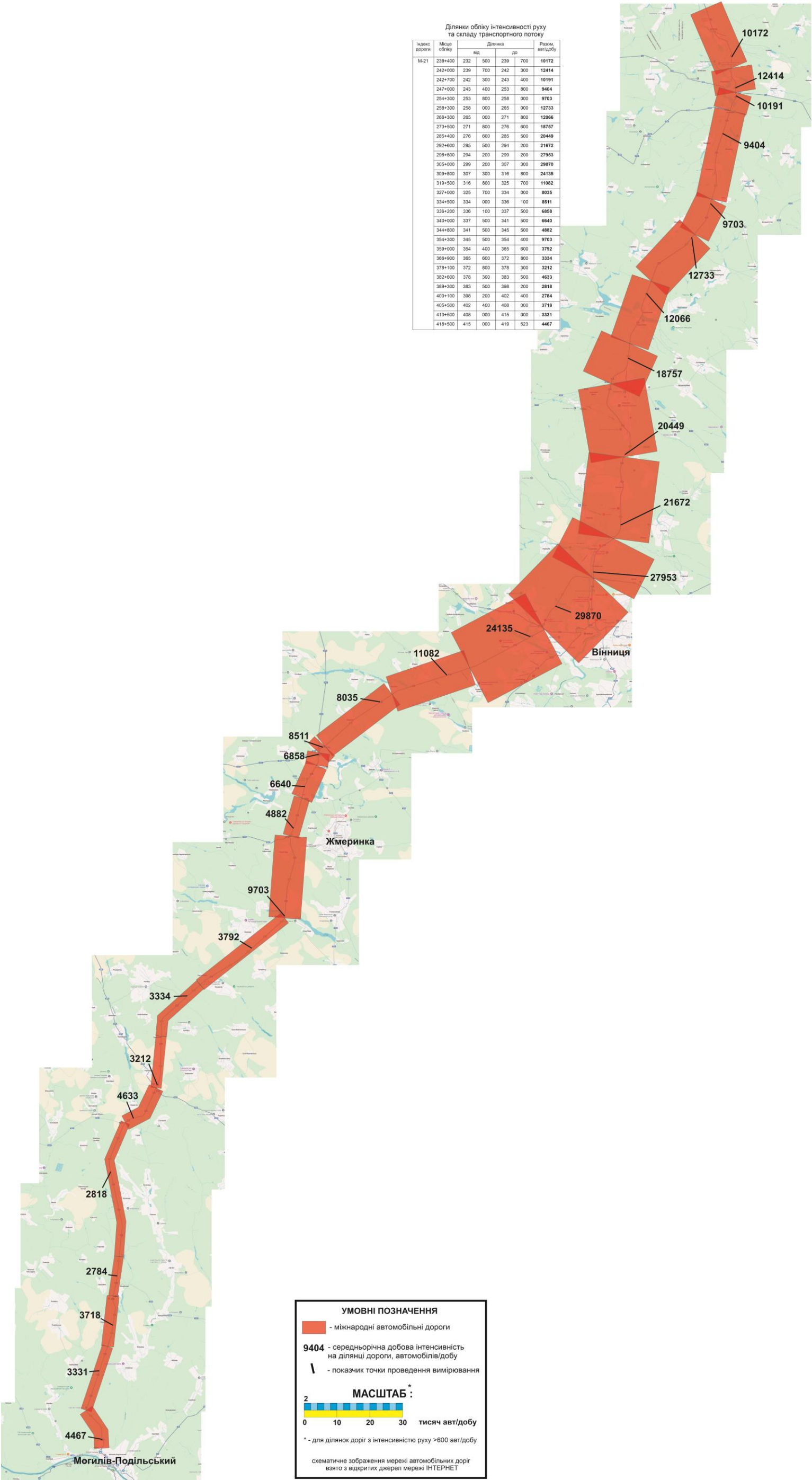
Епюра середньорічної добової інтенсивності руху на основних перегонах автомобільної дороги М-21 Виступовичі - Житомир - Могилів-Подільський (через м. Вінницю) у Вінницькій області
