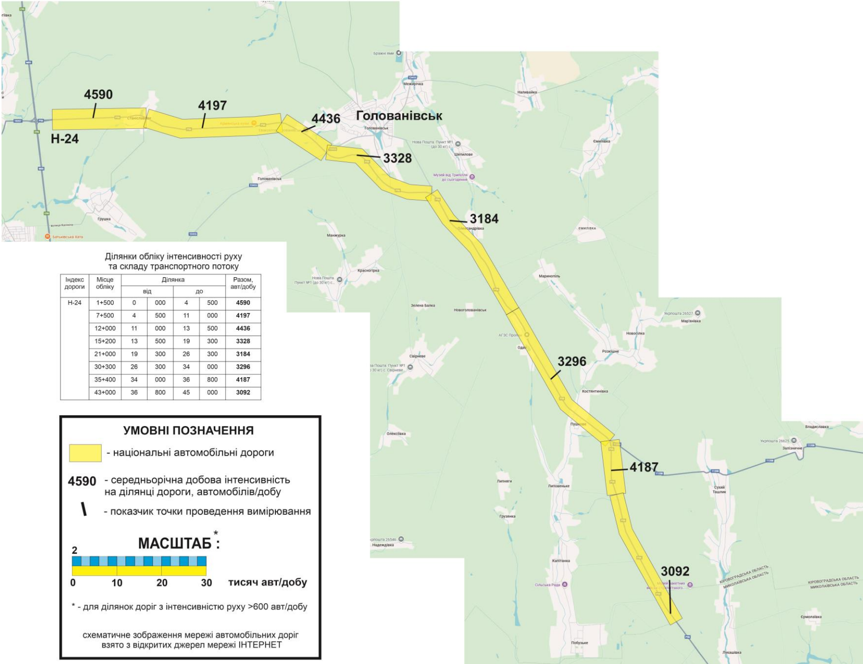
Епюра середньорічної добової інтенсивності руху на основних перегонах автомобільної дороги Н-24 Благівіщенське-Миколаїв (через м. Вознесенськ) у Кіровоградській області
